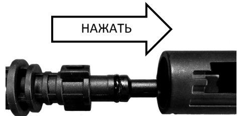
Рис. 5 Подсоединение струйной трубки к пистолету НР6140
